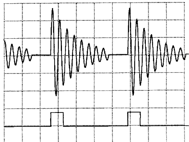
Bild 4: getriggertes Arbitrary-Signal
